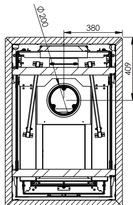
SECTION D-D SCALE 1 : 15
