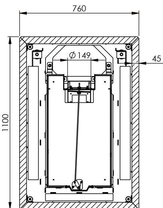
SECTION B-B SCALE 1 : 15
