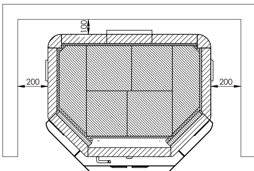
SECTION A-A SCALE 1 : 15
