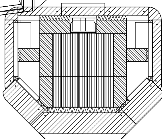
SECTION 6-6 SCALE 1 : 15
