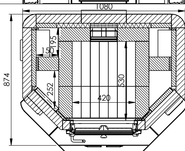
SECTION B-B SCALE 1 : 15
