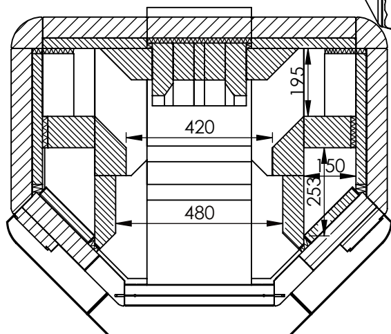
SECTION 5-5 SCALE 1 : 15
