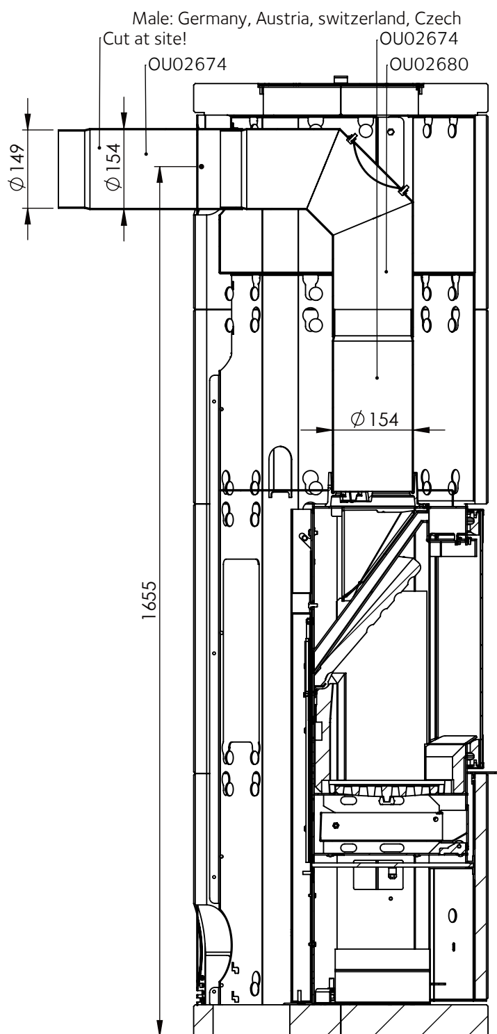
SECTION B-B SCALE 1 : 10
