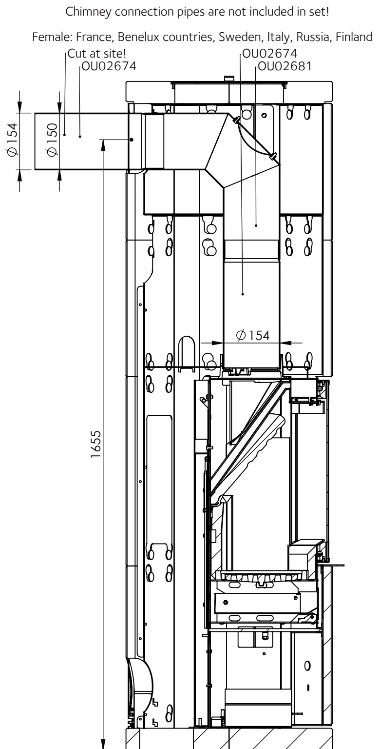
SECTION A-A SCALE 1 : 10
