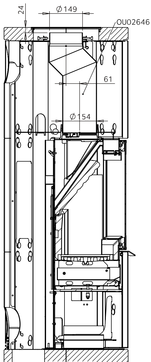
SECTION D-D SCALE 1 : 10
