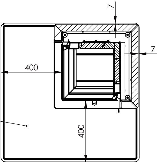
SECTION AK-AK SCALE 1 : 15
