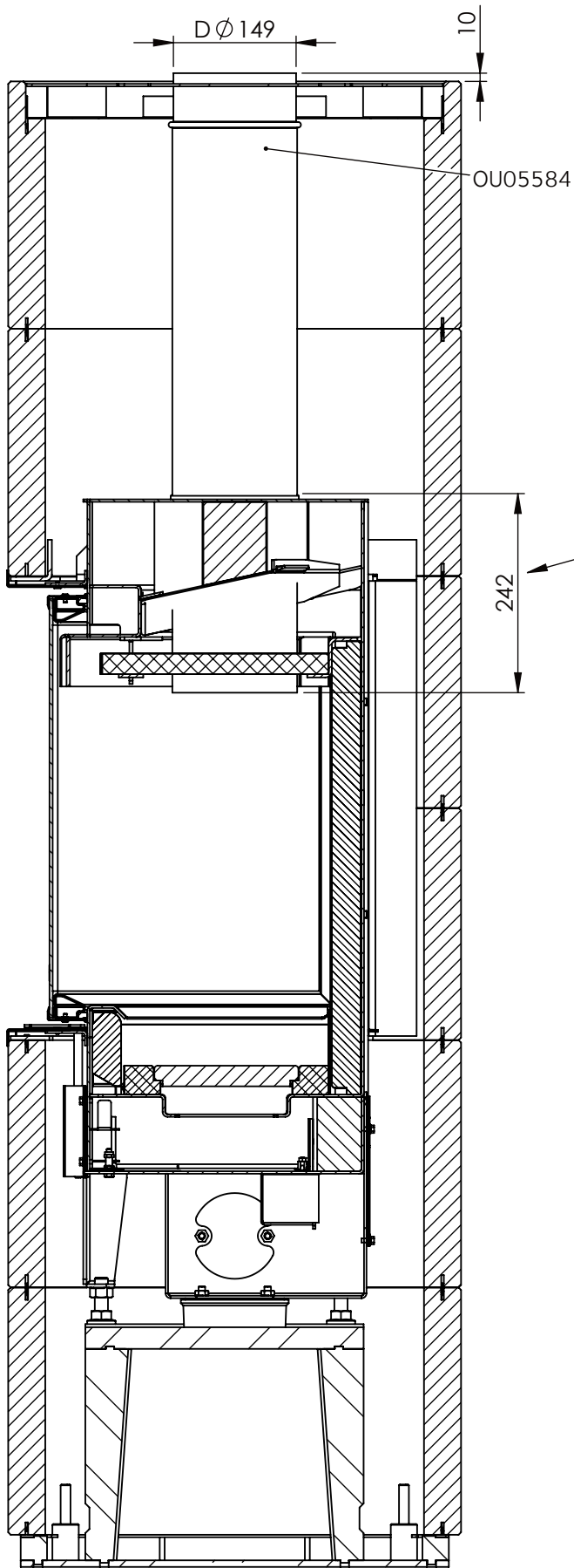
SECTION V-V SCALE 1 : 8
